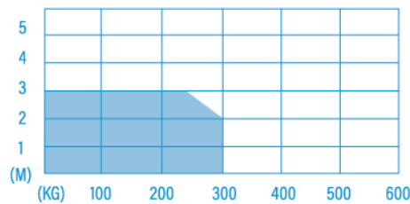
PW 320/320K
